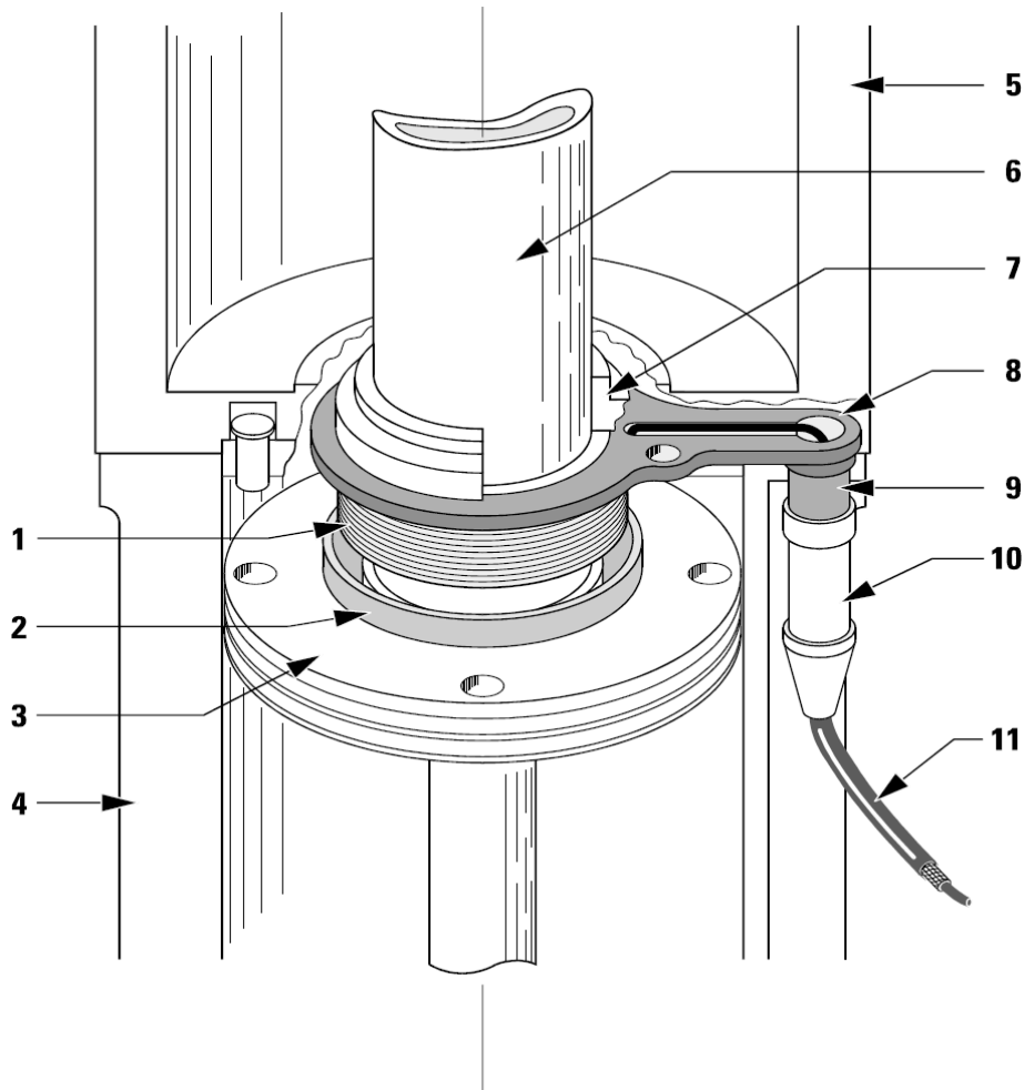
Bild 6: Sensor im Pegelmechanismus
