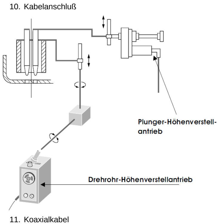
Bild 7: Mechanischer Speiser mit Plunger- und Drehrohr-Höhenverstellung
