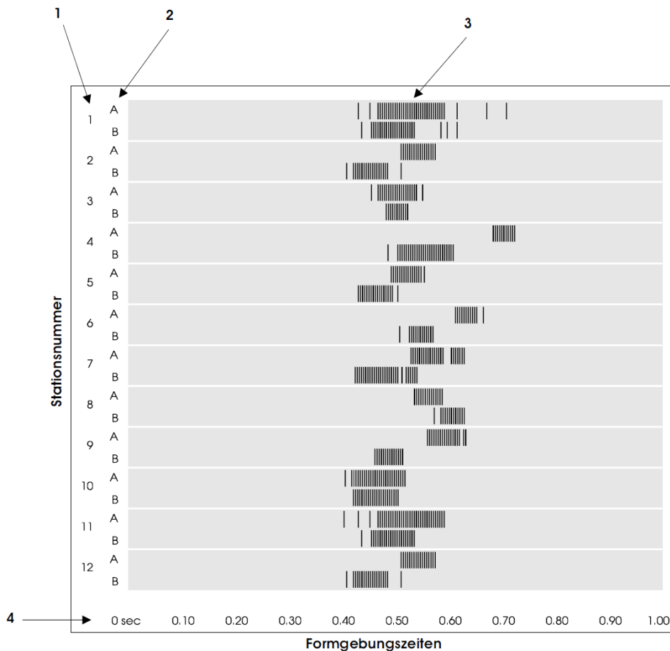
Bild 2: Preßzeit (Stempelverweilzeit)
